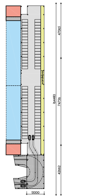
mezzanine/parkeerdek
